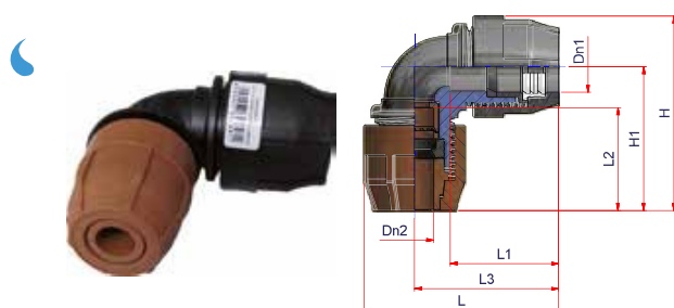
GOMITO TRANSIZIONE TRANSITION ELBOW
