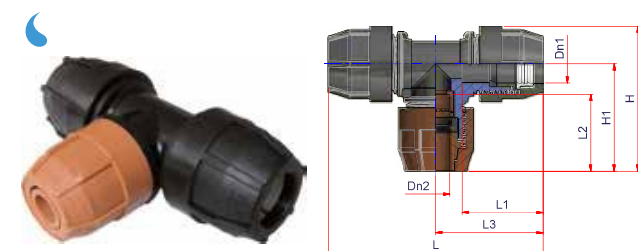
TEE TRANSIZIONE TRANSITION TEE
