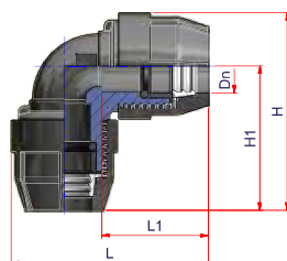
GOMITO 90° 90° ELBOW
