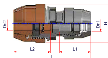
MANICOTTO TRANSIZIONE TRANSITION COUPLER
