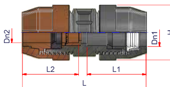
MANICOTTO TRANSIZIONE TRANSITION COUPLER
