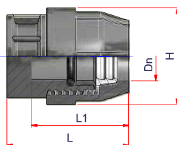
TAPPO END CAP
